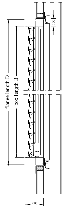
LONGITUDINAL CROSS SECTION
